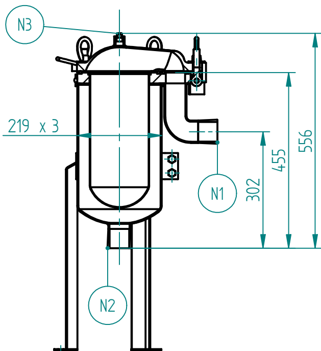
Schnitt A-A
